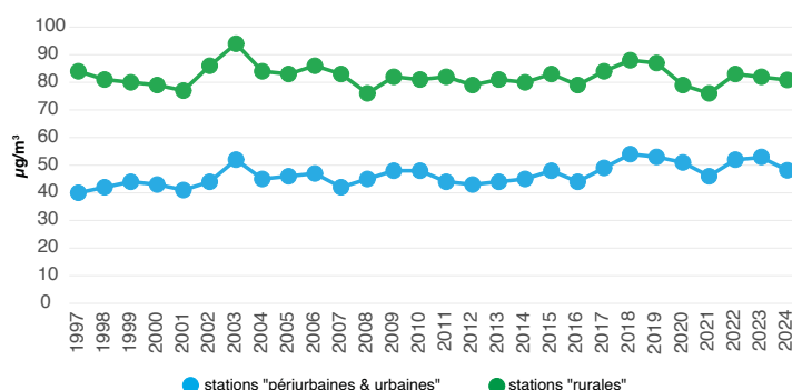
Moyennes des concentrations d'ozone troposphérique (mesurées pour des stations de typologies rurales et urbaines/péri-urbaines)
