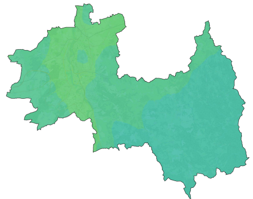
Particules - PM_{2.5} Moyenne annuelle en \mu g/m^3
