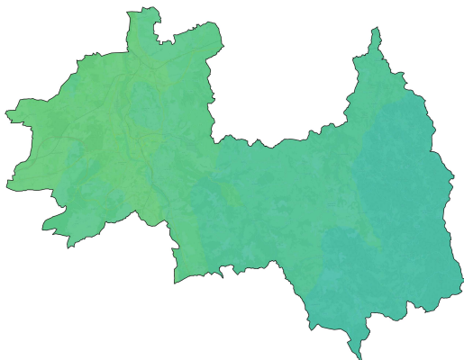
Particules - PM_{10} Moyenne annuelle en \mu g/m^3
