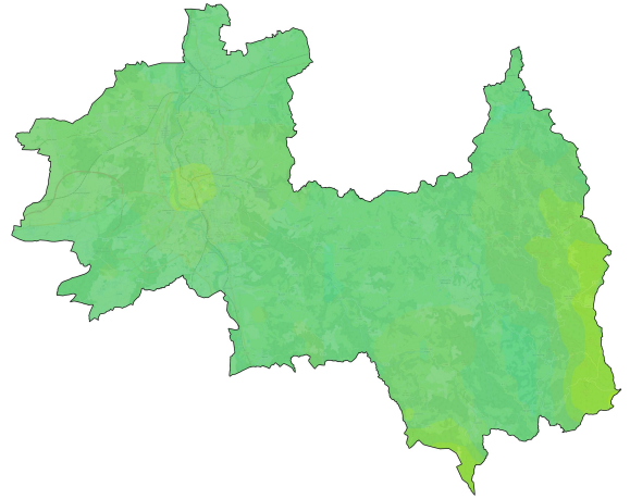
Ozone - O_3 Nb de jours avec dépassement de 120 \mu g/m^3 sur 8h
