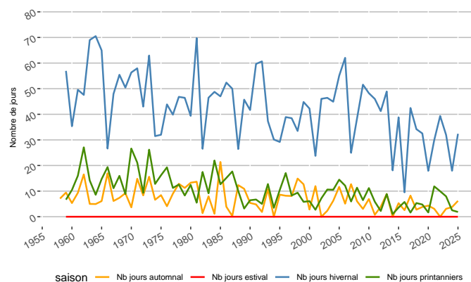
Évolution du nombre de jours de gel saisonnier
