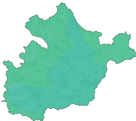
Particules - PM_{10} Moyenne annuelle en \mu g/m^3
