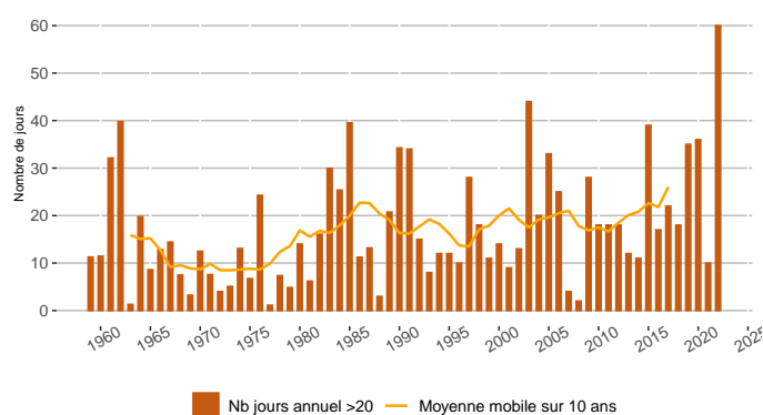
Évolution du nombre annuel de jours où l'Indice Feu Météo > 20 dans le département : Haute-Loire
