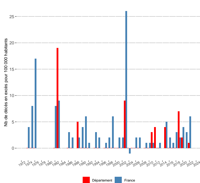
Évolution des taux de décès en excès pendant les périodes de canicule - Haute-Loire (1974-2019)
