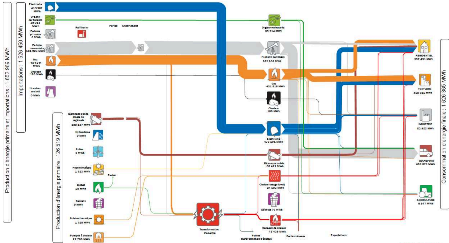
Flux d'énergie 2021 CA Annemasse-Les Voirons-Agglomération
