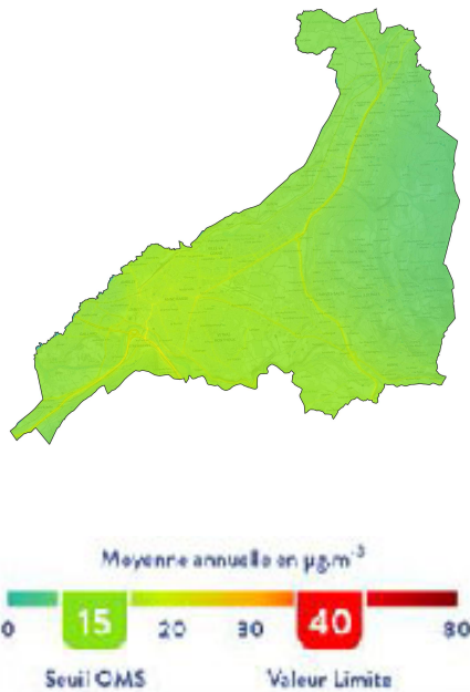
Particules - PM_{10} Moyenne annuelle en \mu\text{g}/\text{m}^3
