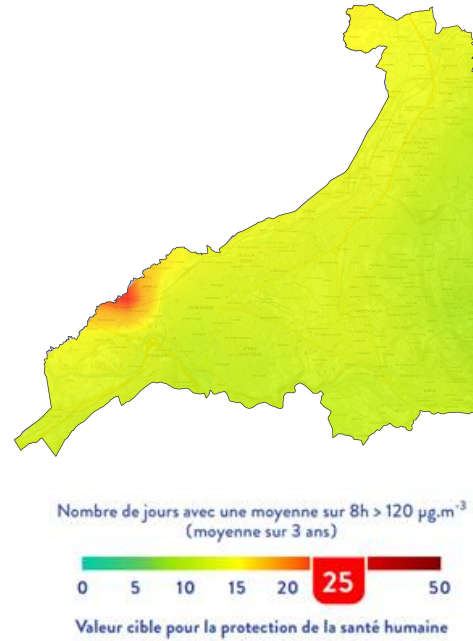
Ozone - O_3 Nb de jours avec dépassement de 120 \mu\text{g}/\text{m}^3 sur 8h
