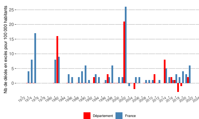
Évolution des taux de décès en excès pendant les périodes de canicule - Haute-Savoie (1974-2019)
