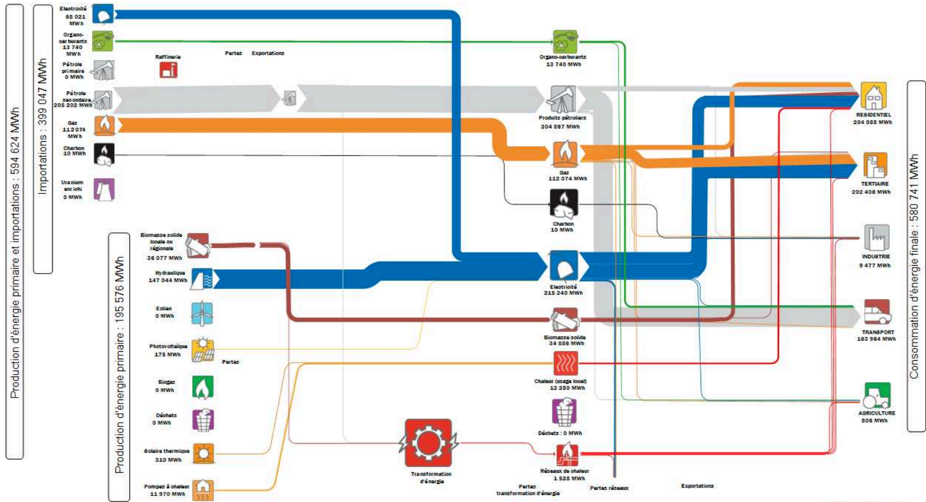
Flux d'énergie 2021 CC de la Vallée de Chamonix-Mont-Blanc
