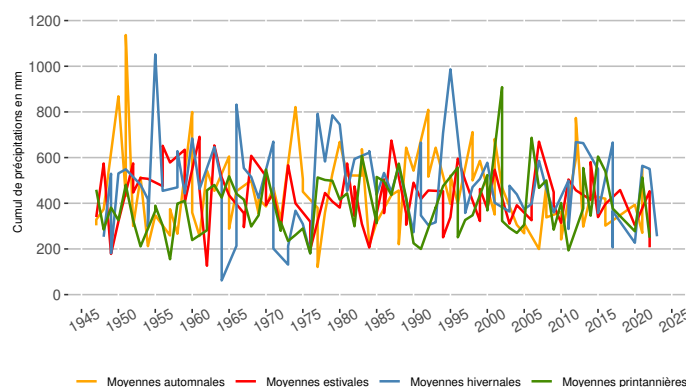
Évolution des cumuls saisonniers de précipitations à Thônes (mm, altitude 630 m)
