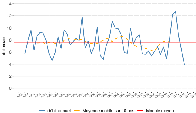
Évolution des débits moyens annuels de La Bourbre à Tignieu-Jamezyieu
