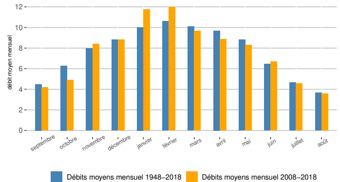
Tendances mensuelles des débits La Bourbre à Tignieu-Jamezyieu
