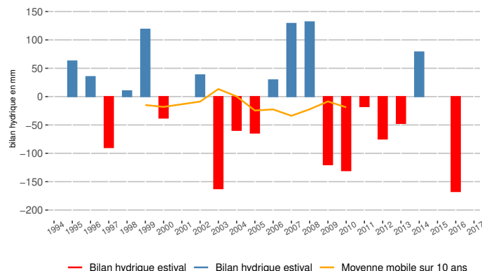
Évolution du bilan hydrique estival à Meythet (1994-2017, juill - sept, mm, altitude 455 m)
