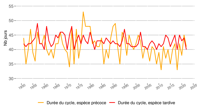
Durée de présence des épis à la station de Lyon-Bron
