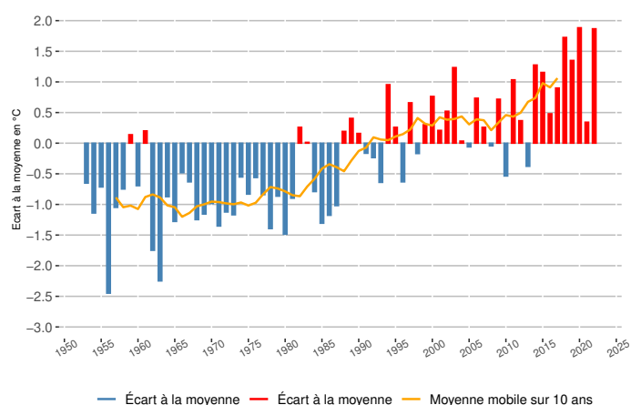
Écart à la moyenne 1981 - 2010 de la température moyenne annuelle à Lyon-Bron (°C, altitude 197 m)
