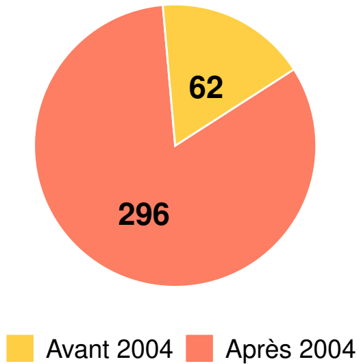
Répartition du nombre de communes en arrêtés sécheresse dans le département : Rhône entre 1989-2004 et 2004-2020
