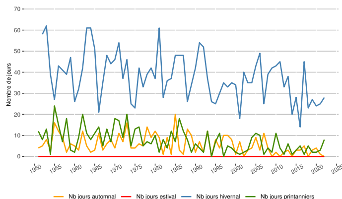
Évolution du nombre de jours de gel saisonnier à Lyon-Bron (altitude 197 m)
