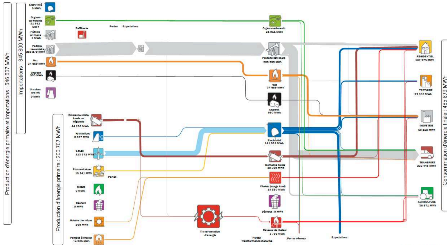
Flux d'énergie 2021 CC Hautes Terres
