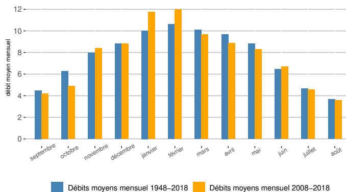
Tendances mensuelles des débits La Bourbre à Tignieu-Jameyzieu
