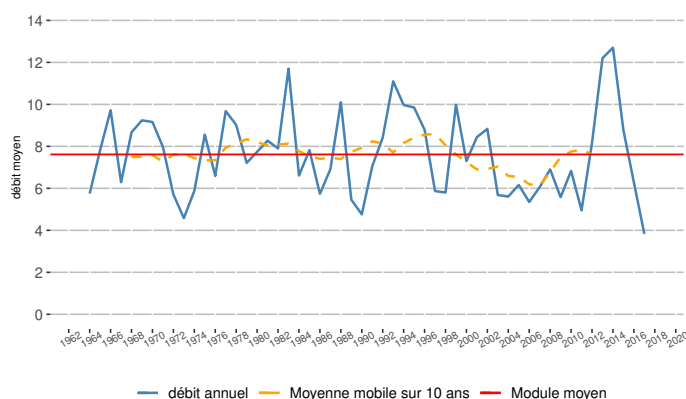
Évolution des débits moyens annuels de La Bourbre à Tignieu-Jameyzieu
