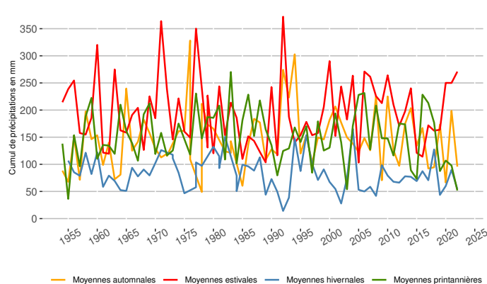
Évolution des cumuls saisonniers de précipitations à Clermont-Ferrand (mm, altitude 331 m)
