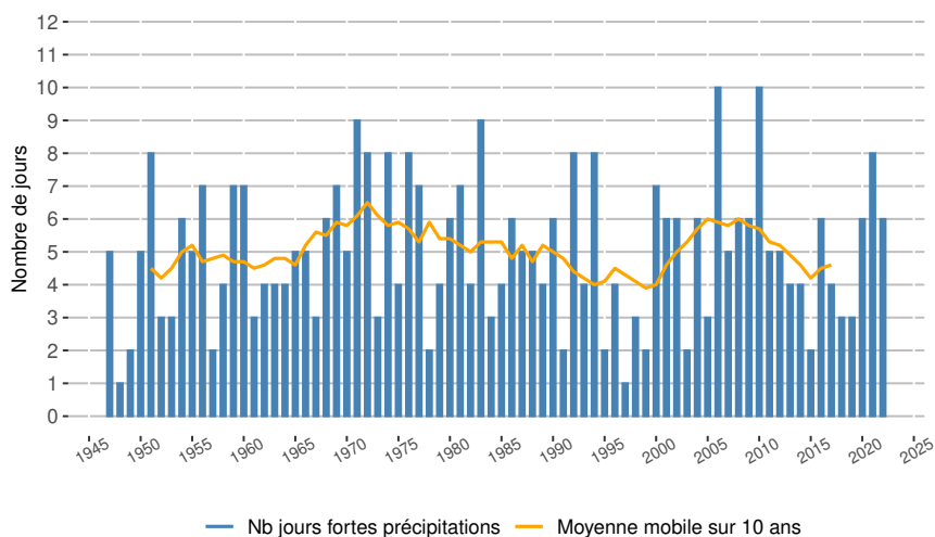
Évolution du nombre de jours de fortes pluies à Clermont-Ferrand (altitude 331 m)
