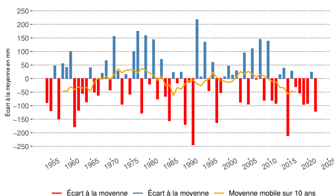
Écart à la moyenne 1981 - 2010 des cumuls annuels de précipitations à Clermont-Ferrand (mm, altitude 331m)
