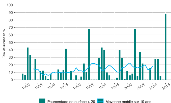
Évolution de la superficie départementale où l'Indice Feu Météo > 20 pendant au moins 20 jours dans le département : Puy-de-Dôme
