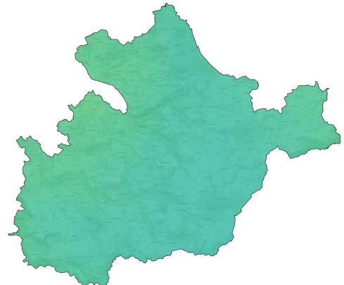
Particules - PM2.5 Moyenne annuelle en \mu g/m^3
