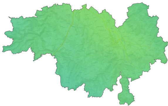
Particules - PM_{10} Moyenne annuelle en \mu g/m^3
