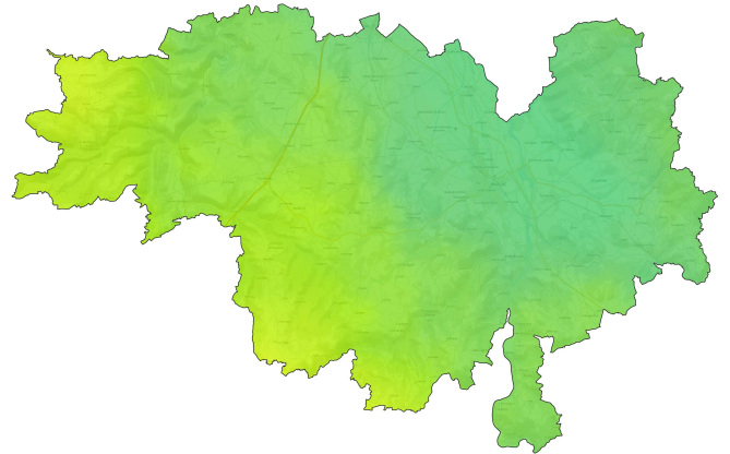
Ozone - O_3 Nb de jours avec dépassement de 120 \mu g/m^3 sur 8h
