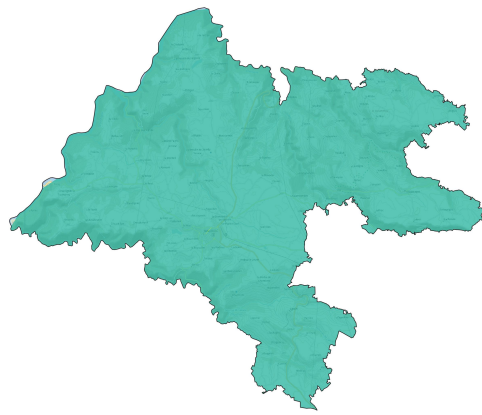
Dioxyde d'azote - NO_2 Moyenne annuelle en \mu\text{g}/\text{m}^3
