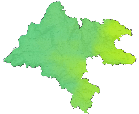
Ozone - O_3 Nb de jours avec dépassement de 120 \mu\text{g}/\text{m}^3 sur 8h
