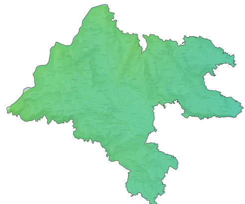
Particules - PM_{2.5} Moyenne annuelle en \mu\text{g}/\text{m}^3
