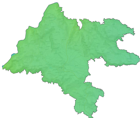
Particules - PM_{10} Moyenne annuelle en \mu\text{g}/\text{m}^3
