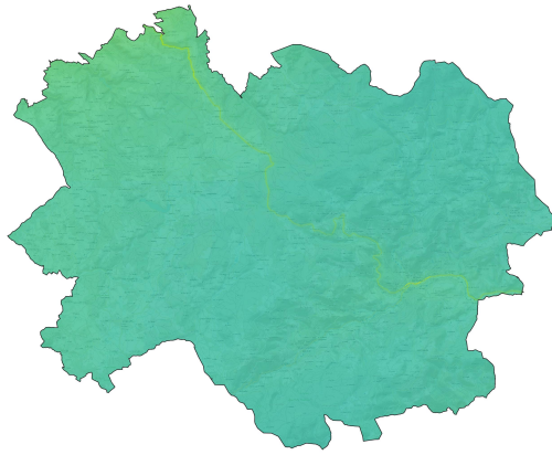
Dioxyde d'azote - NO_2 Moyenne annuelle en \mu\text{g}/\text{m}^3
