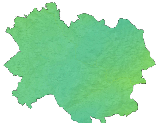
Particules - PM_{2.5} Moyenne annuelle en \mu\text{g}/\text{m}^3
