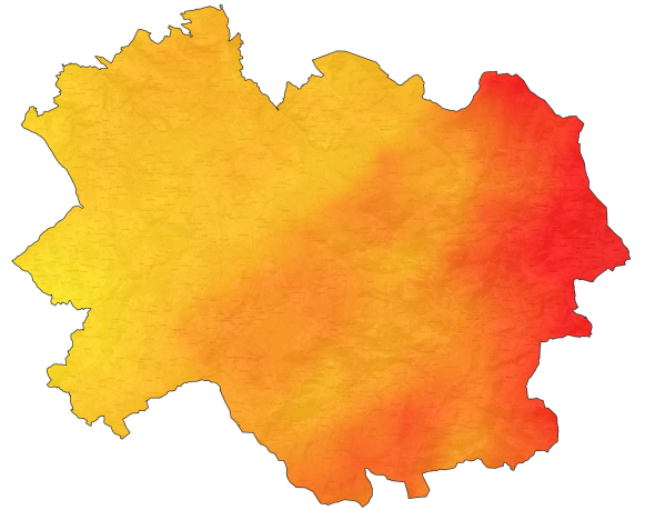
Ozone - O_3 Nb de jours avec dépassement de 120 \mu\text{g}/\text{m}^3 sur 8h
