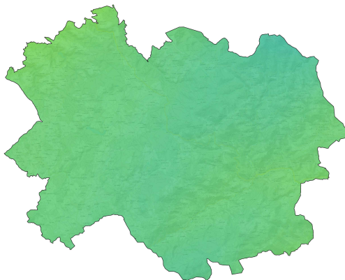
Particules - PM_{10} Moyenne annuelle en \mu\text{g}/\text{m}^3
