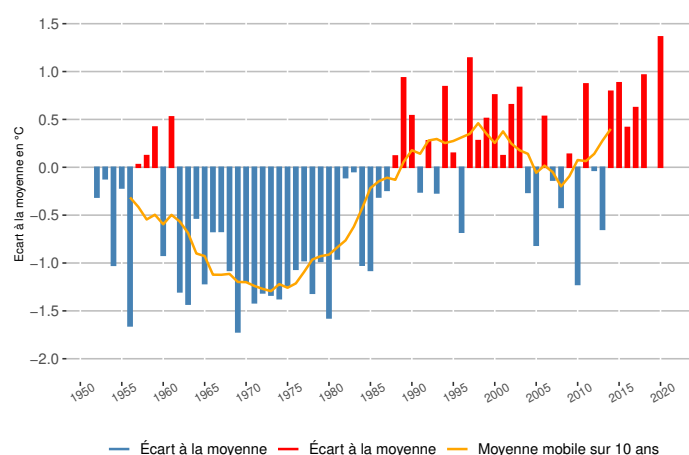
Écart à la moyenne 1981 - 2010 de la température moyenne annuelle à Issanlas (°C, altitude 1209 m)
