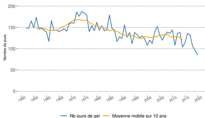
Évolution du nombre de jours de gel annuels à Issanlas (altitude 1209 m)
