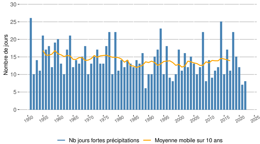
Évolution du nombre de jours de fortes pluies à Issanlas (altitude 1209 m)
