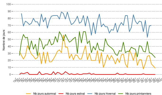
Évolution du nombre de jours de gel saisonnier à Issanlas (altitude 1209 m)
