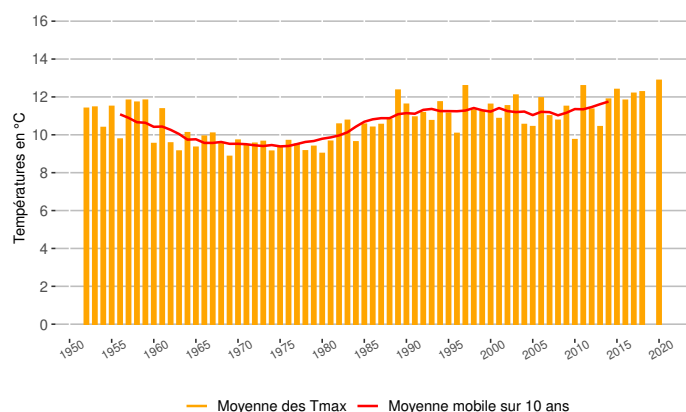
Évolution des températures maximales annuelles à Le Puy-Chadrac (°C, altitude 714 m)
