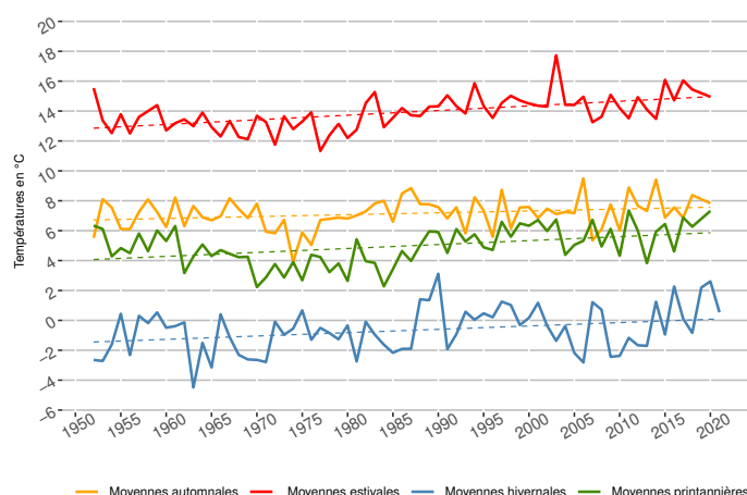
Évolution des températures moyennes saisonnières à Issanlas (°C, altitude 1209 m)
