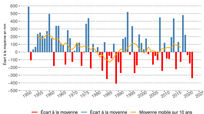
Écart à la moyenne 1981 - 2010 des cumuls annuels de précipitations à Issanlas (mm, altitude 1209m)
