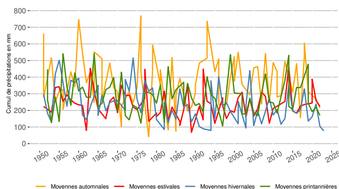
Évolution des cumuls saisonniers de précipitations à Issanlas (mm, altitude 1209 m)
