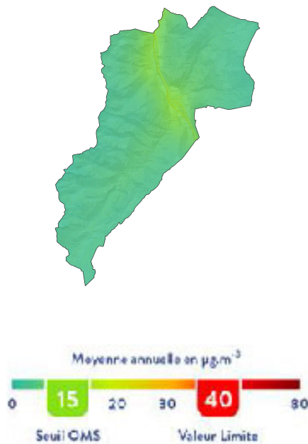
Particules - PM_{10} Moyenne annuelle en \mu\text{g}/\text{m}^3
