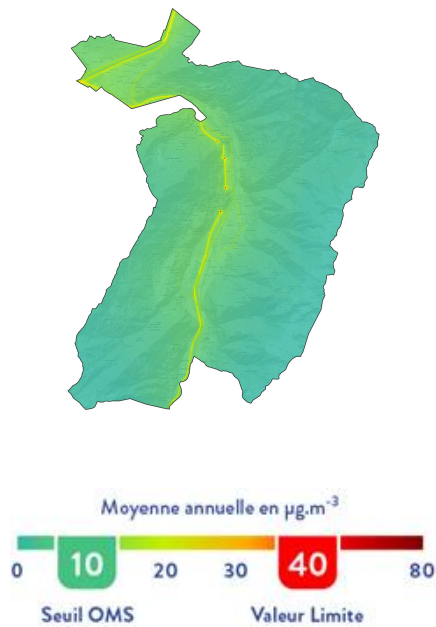
Dioxyde d'azote - NO_2 Moyenne annuelle en \mu\text{g}/\text{m}^3
