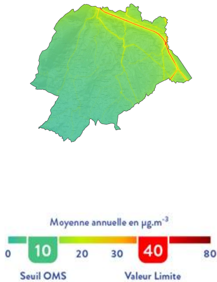
Particules - PM_{10} Moyenne annuelle en \mu\text{g}/\text{m}^3
