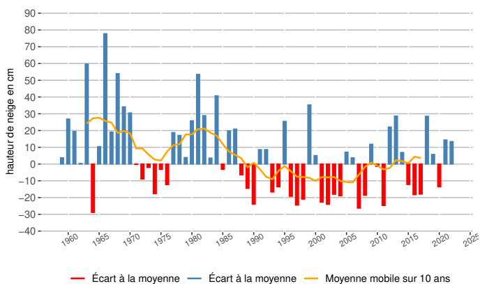
Écart à la moyenne 1981-2010 de la hauteur de neige moyenne à Chamonix (cm, altitude 1042 m)
