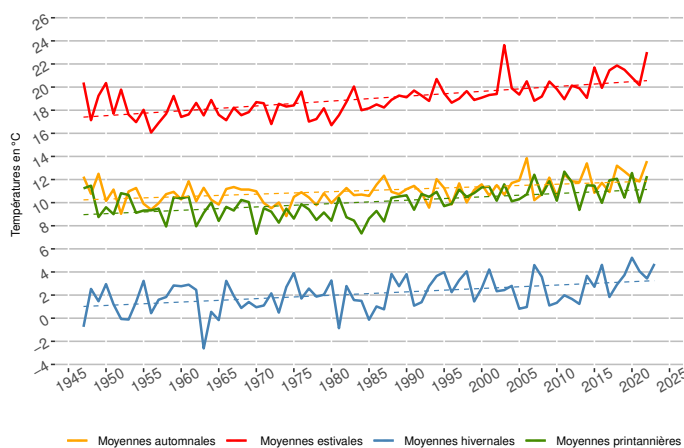
Évolution des températures moyennes saisonnières à Cran-Gevrier (°C, altitude 426 m)
