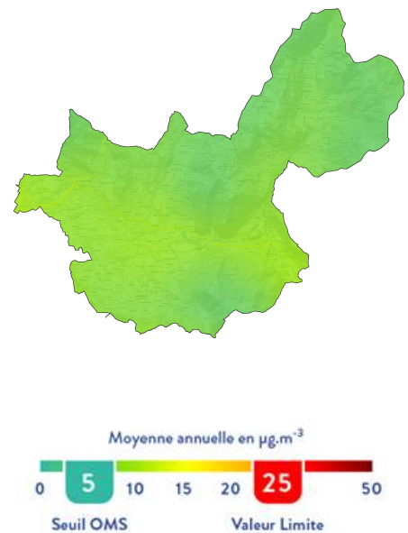
Particules - PM_{2.5} Moyenne annuelle en \mu\text{g}/\text{m}^3
