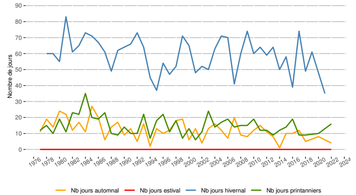
Évolution du nombre de jours de gel saisonnier à Cran-Gevrier (altitude 426 m)
