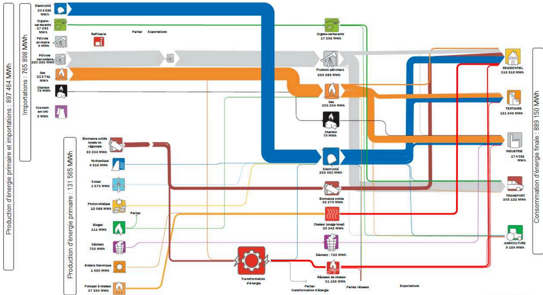
Flux d'énergie 2021 TEPOS-CV CC du Bassin d'Aubenas
