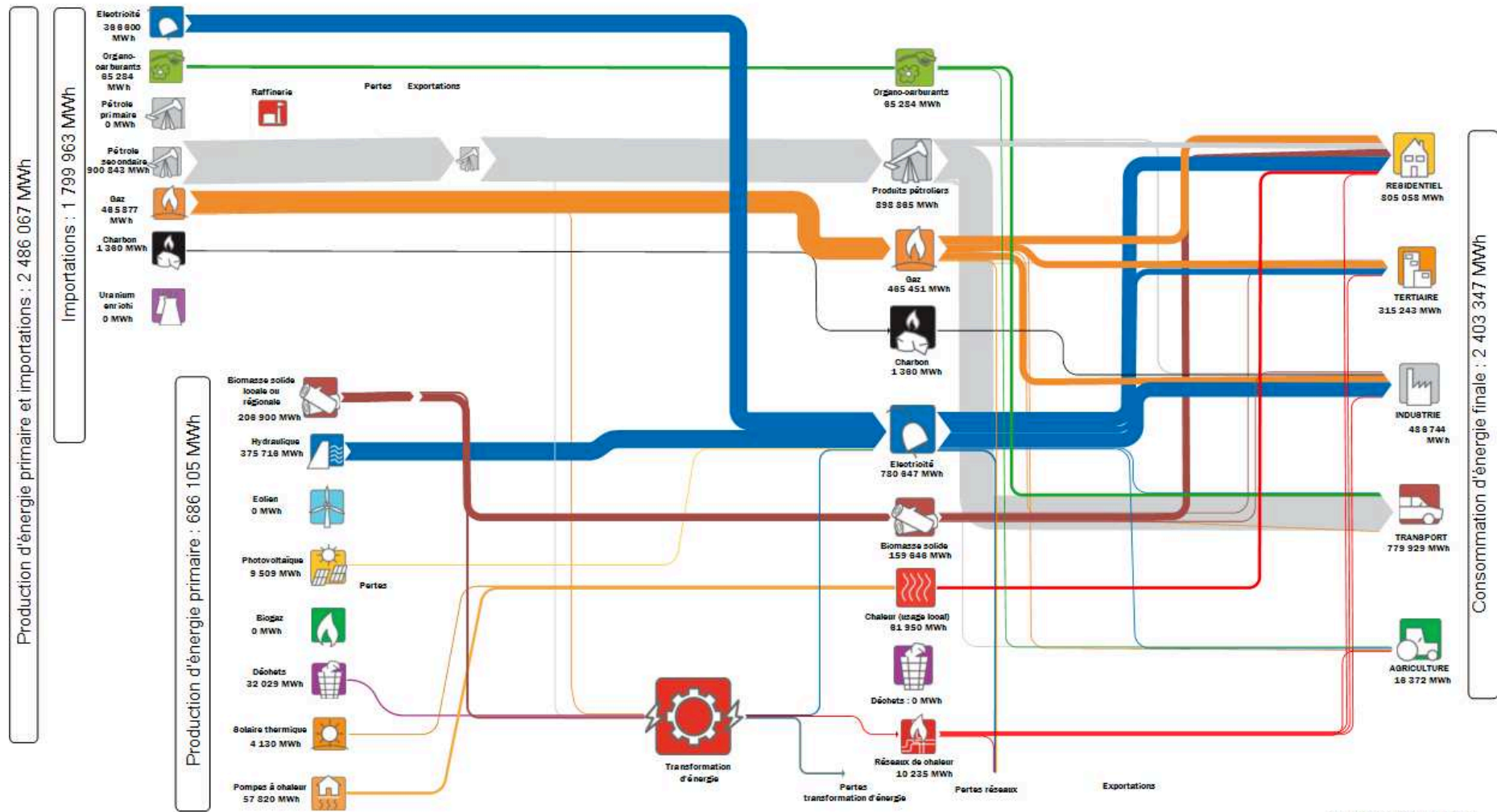
Flux d'énergie 2021 TEPOS-CV CC Le Grésivaudan
