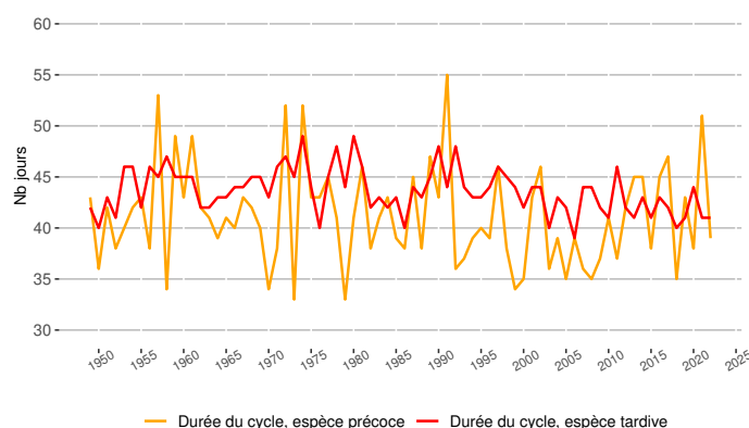
Durée de présence des épis à la station de Bourg-Saint-Maurice
