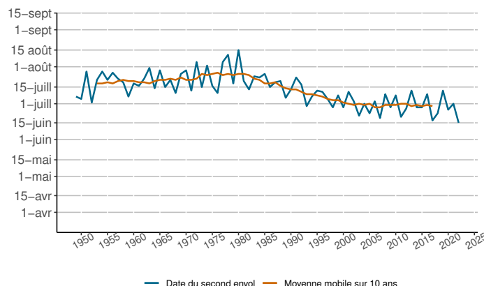
Date de second envol du scolyte à la station de Bourg-Saint-Maurice
