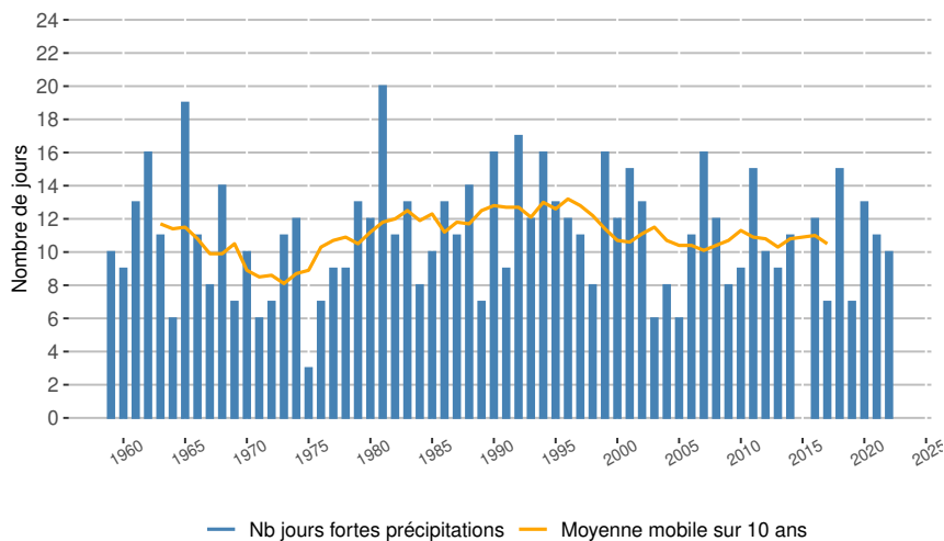
Évolution du nombre de jours de fortes pluies à Bourg-Saint-Maurice (altitude 865 m)
