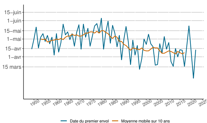
Date de premier envol du scolyte à la station de Bourg-Saint-Maurice
