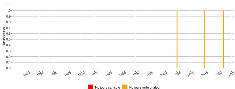
Évolution du nombre de jours de canicule et de forte chaleur à Bourg-Saint-Maurice (altitude 865 m)
