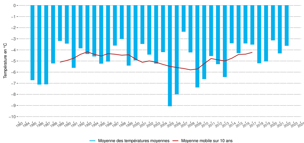
Évolution des températures moyennes sur la saison hivernale à Bessans (20 déc - 20 mars, °C, altitude 1715 m)
