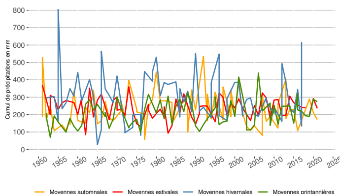
Évolution des cumuls saisonniers de précipitations à Bourg-Saint-Maurice (mm, altitude 865 m)
