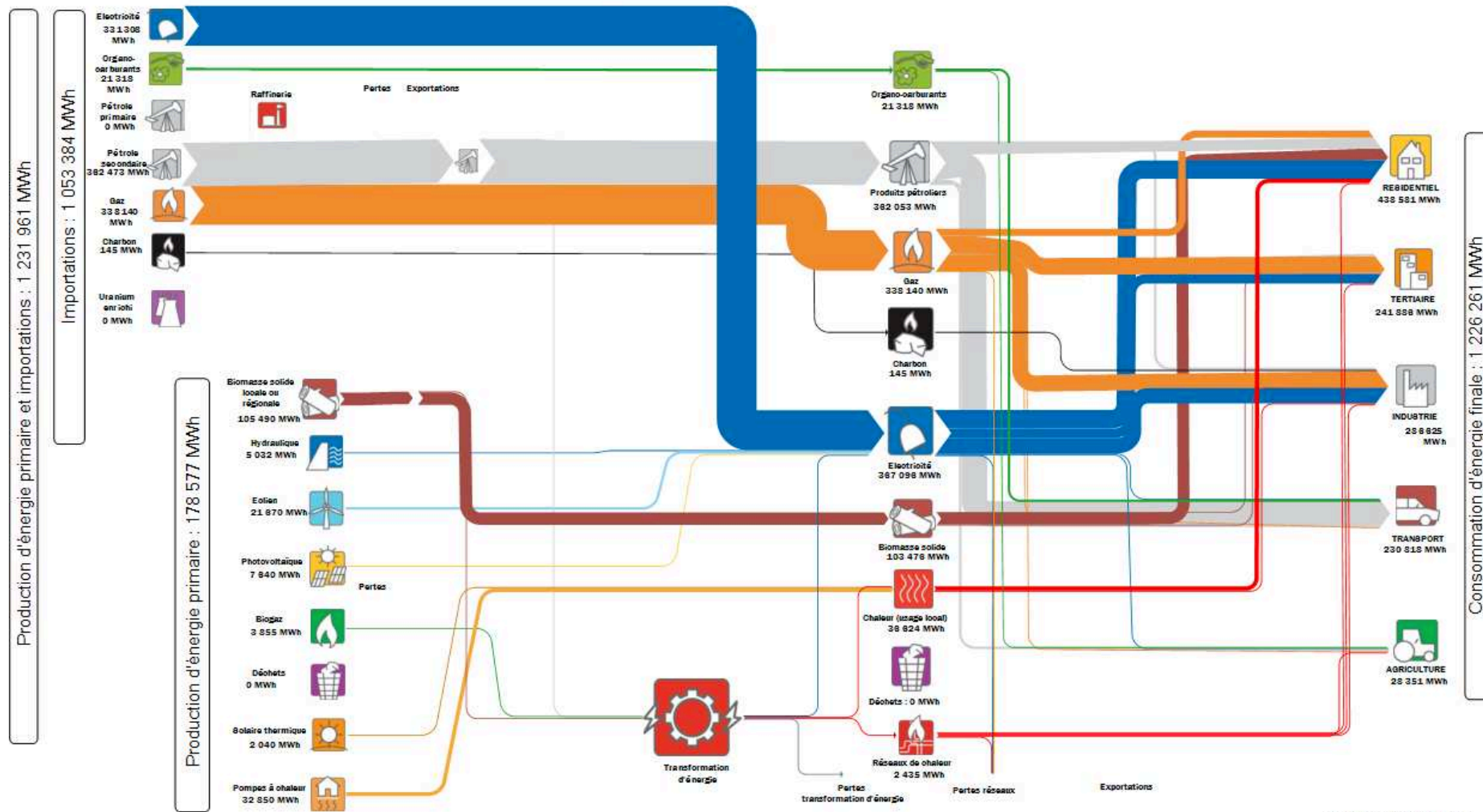
Flux d'énergie 2021 TEPOS-CV CA Annonay-Rhône + CC Val d'Ay
