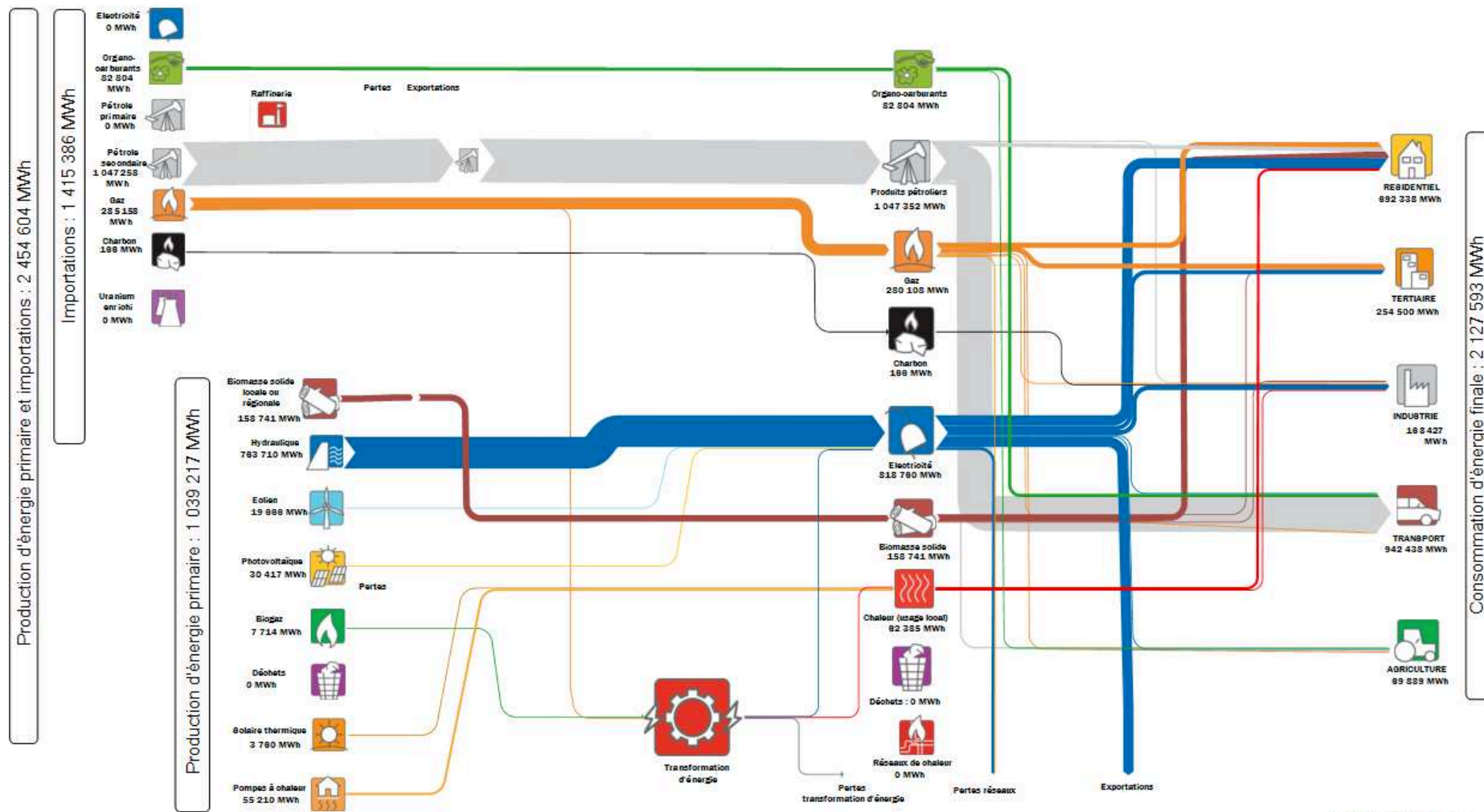
Flux d'énergie 2021 TEPOS-CV Arche Agglo Rhône Crussol
