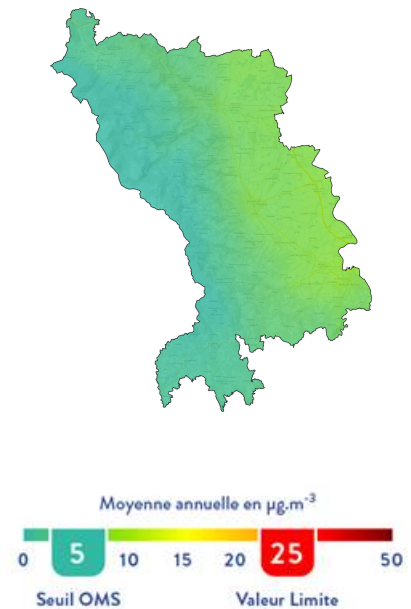
Particules - PM_{2.5} Moyenne annuelle en \mu\text{g}/\text{m}^3
