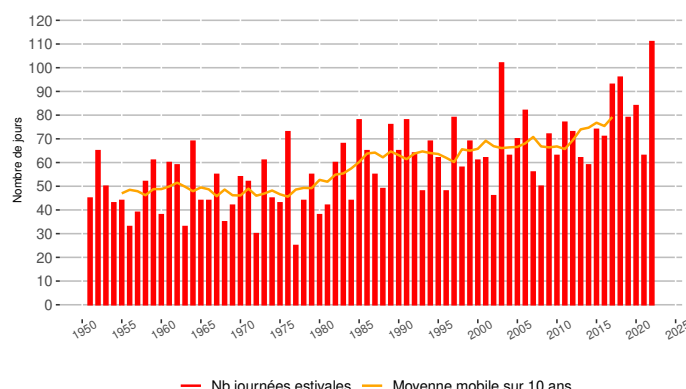
Évolution du nombre de journées estivales à Saint-Etienne-Bouthéon (°C, altitude 395 m)
