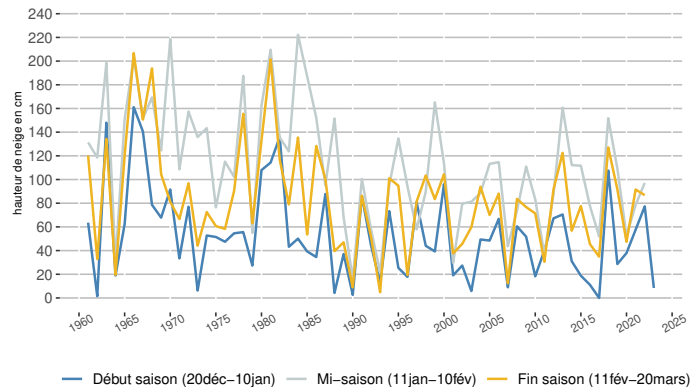
Évolution de la hauteur de neige moyenne à Col de Porte (cm, altitude 1325 m)
