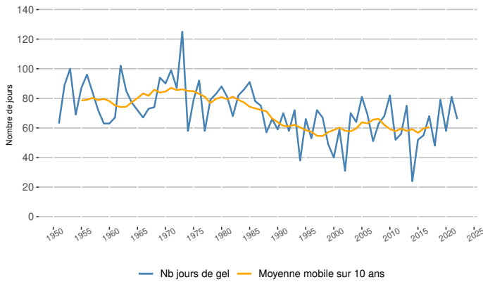
Évolution du nombre de jours de gel annuels à Saint-Etienne-Bouthéon (altitude 395 m)
