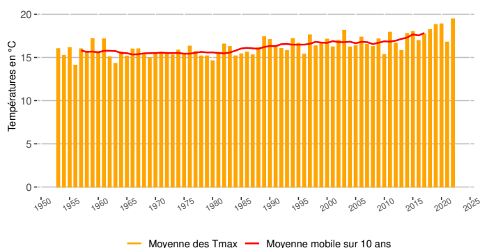
Évolution des températures maximales annuelles à Saint-Etienne-Bouthéon (°C, altitude 395 m)
