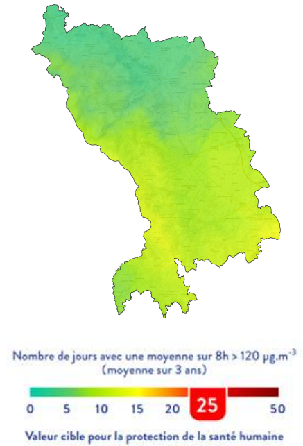
Ozone - O_3 Nb de jours avec dépassement de 120 \mu\text{g}/\text{m}^3 sur 8h
