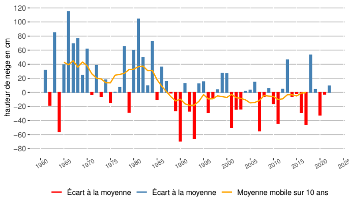
Écart à la moyenne 1981-2010 de la hauteur de neige moyenne à Col de Porte (cm, altitude 1325 m)
