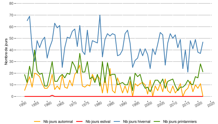
Évolution du nombre de jours de gel saisonnier à Saint-Etienne-Bouthéon (altitude 395 m)
