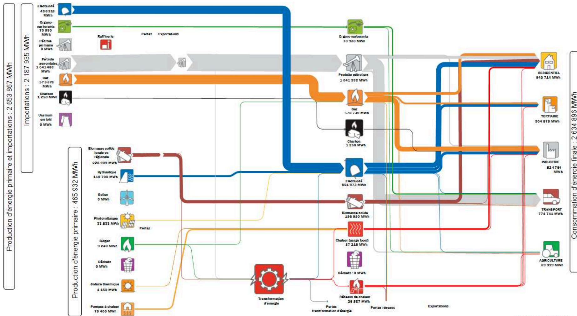
Flux d'énergie 2021 TEPOS-CV CA Loire Forez
