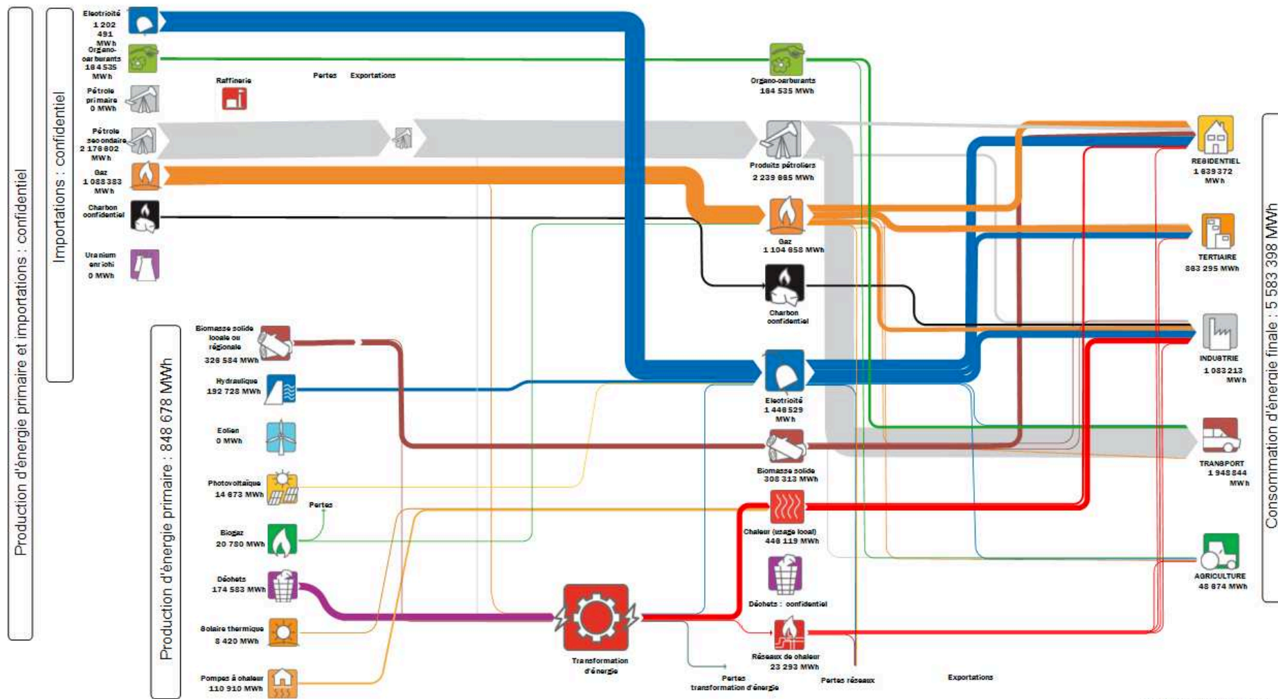
Flux d'énergie 2021 TEPOS-CV CA Pays Voironnais et PNR de la Chartreuse
